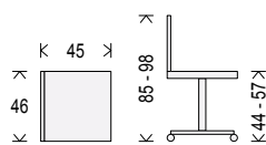
Maße Drehstuhl
