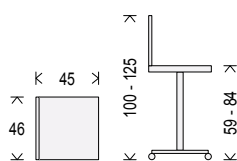
Maße Counterstuhl
