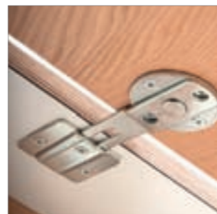
Ansicht von unten Tischplattenverbinder 30224
